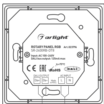
Шина DALI — AC 220 В
